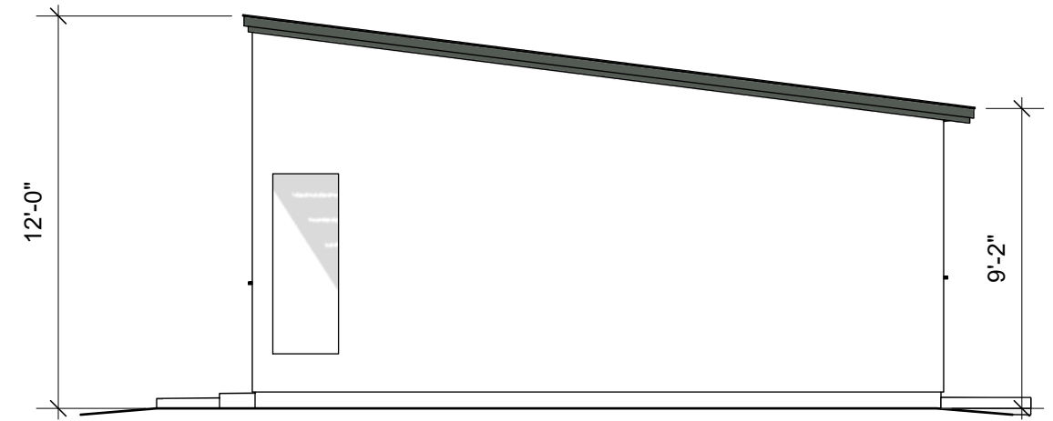
ELEVATION B
