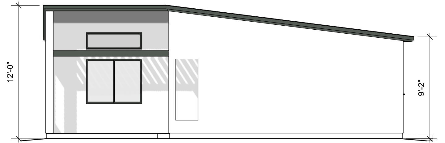
ELEVATION B
