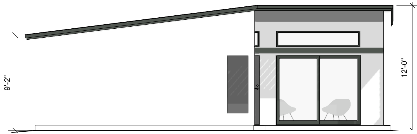
ELEVATION A
