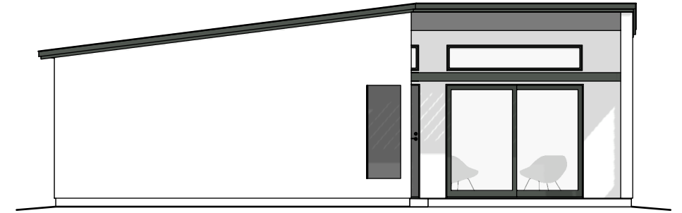
ELEVATION A
